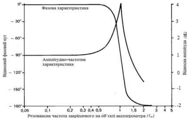
Рисунок 3.7 - Амплітудно-частотна і фазова характеристики п'єзоелектричного акселерометра
