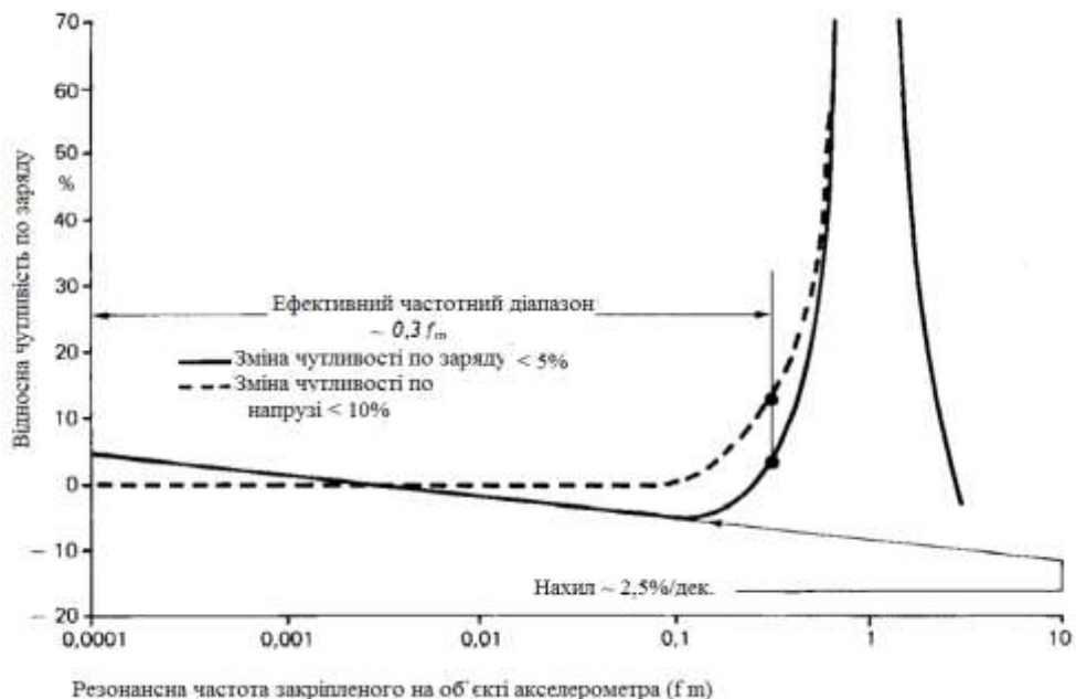
Рисунок 3.4 - Криві залежності чутливості по заряду і напрузі від частоти акселерометра з п'єзоелементом із кераміки
