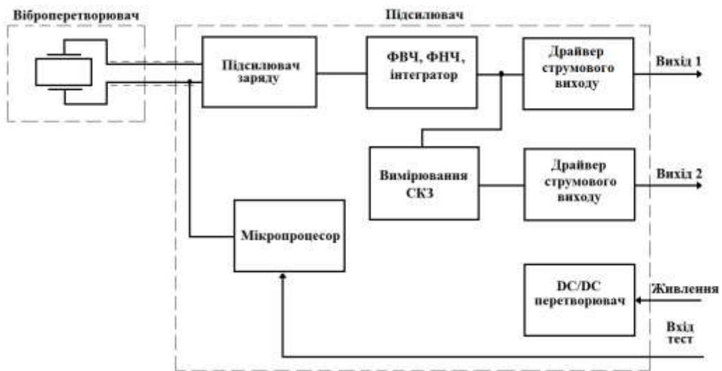
Рисунок 4.2 - Структурна схема
